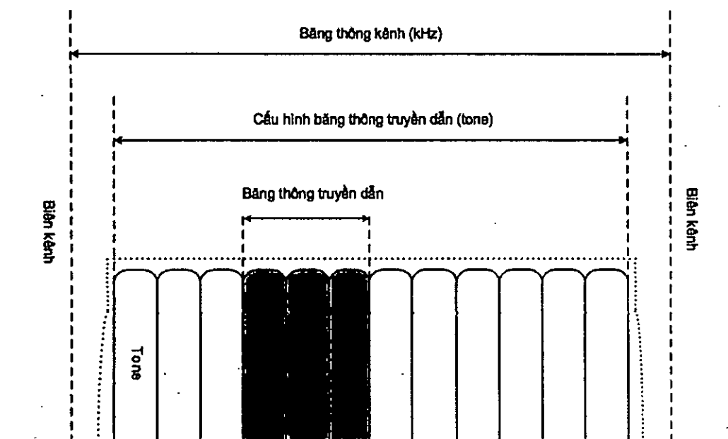
Hình 1 - Băng thông kênh và cấu hình băng thông truyền dẫn NB
